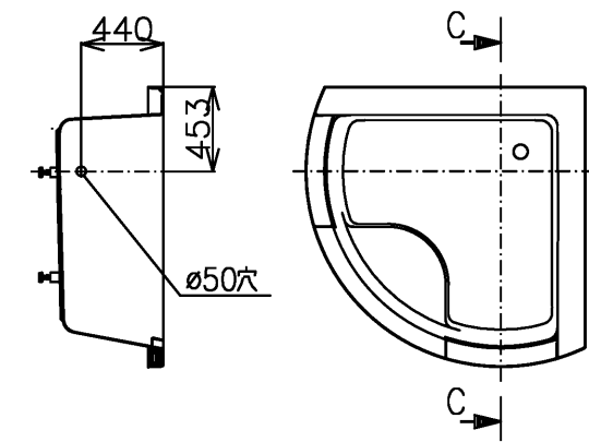
断面C-C 追焚用穴あけ可能位置
